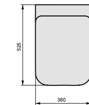
Wc Brio sospeso Wc Brio wall-hung Bidet Brio sospeso Bidet Brio wall-hung
